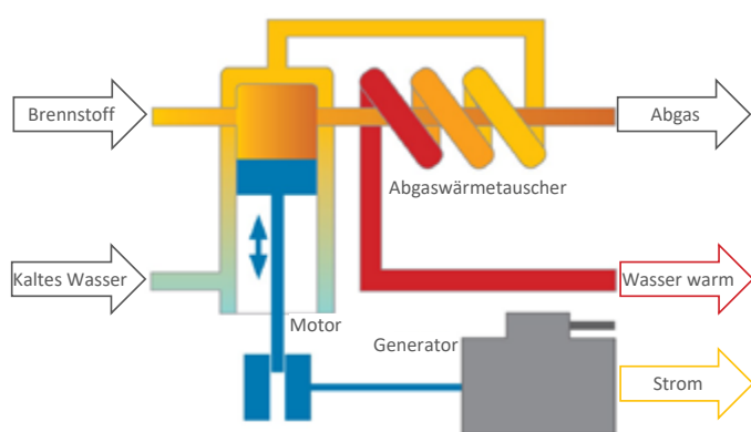
Bild oben: Ein schematische Darstellung der Funktionsweise eines Blockheizkraftwerkes.
